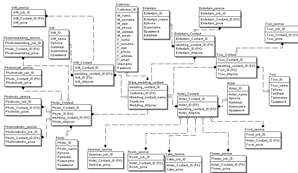
รูปที่ 6-2 แสดงอีอาร์ไดอะแกรมของระบบ Olala Wedding Planner
